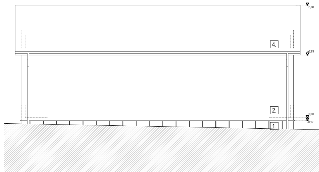
Észak-keleti homlokzat
