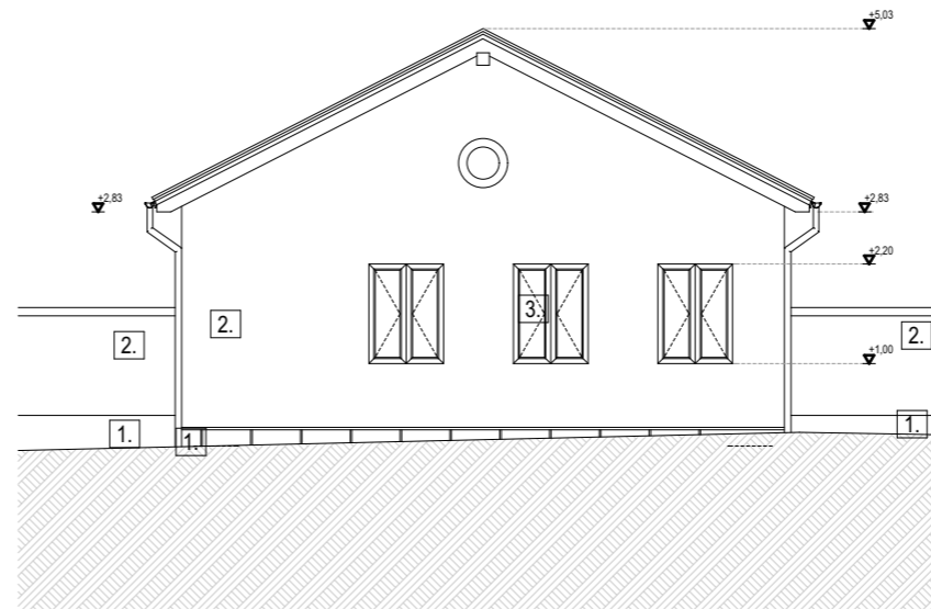
Dél-keleti homlokzat
