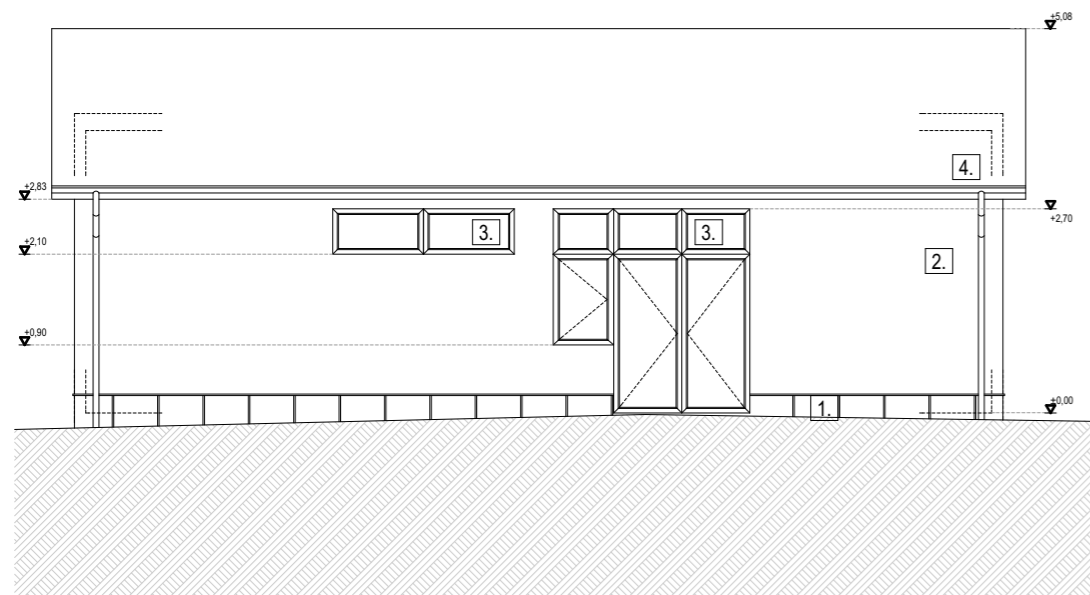
Dél-nyugati homlokzat
