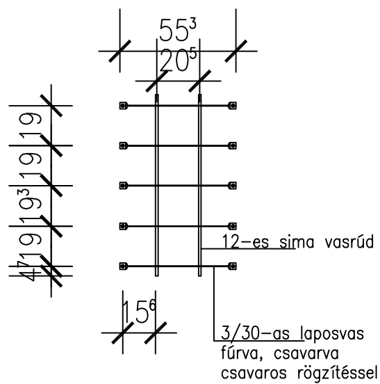
rács terve
