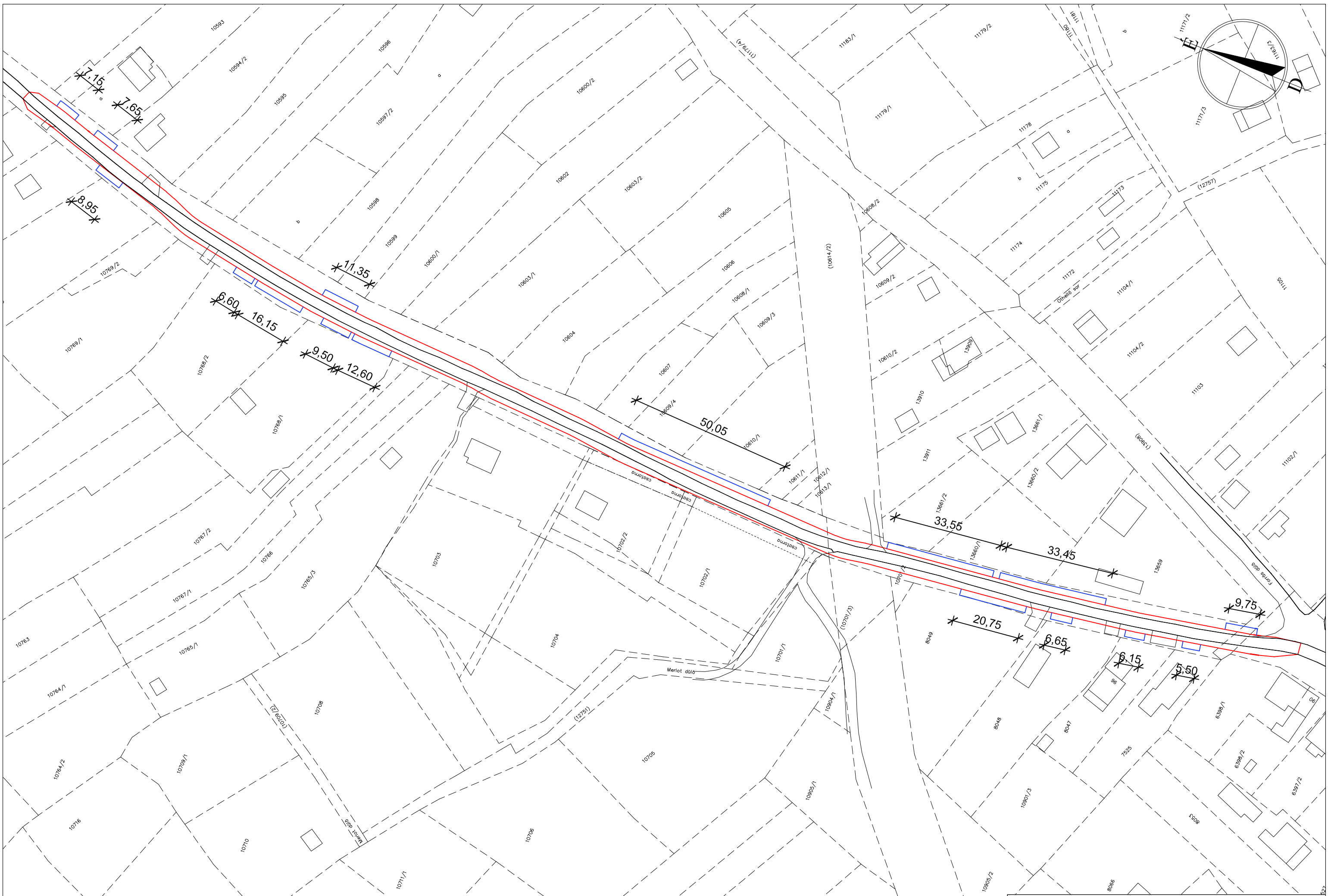
Monor, Strázsahegy szegélyek, parkolók Általános helyszínrajz 3. sz. - Mendei utca 1:1000
