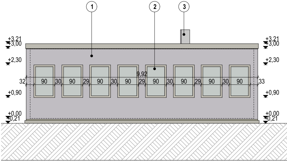
ÉSZAKNYUGATI HOMLOKZAT
