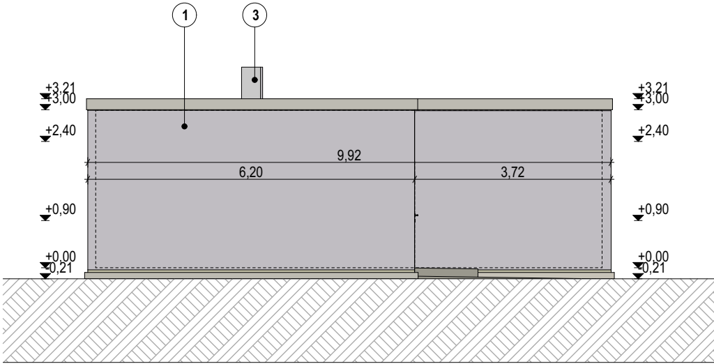
DÉLKELETI HOMLOKZAT
