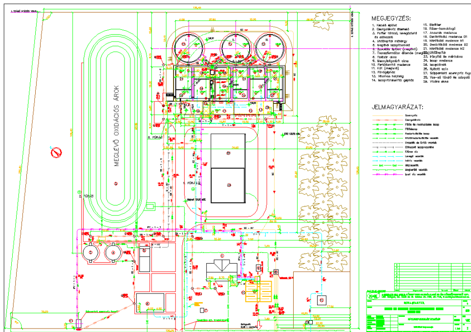
21. ábra: A Monori Szennyvíztisztító Telep helyszínrajza a meglévő műtárgyakkal [Üzemeltetési szabályzat - DAKÖV Kft., 2022]
