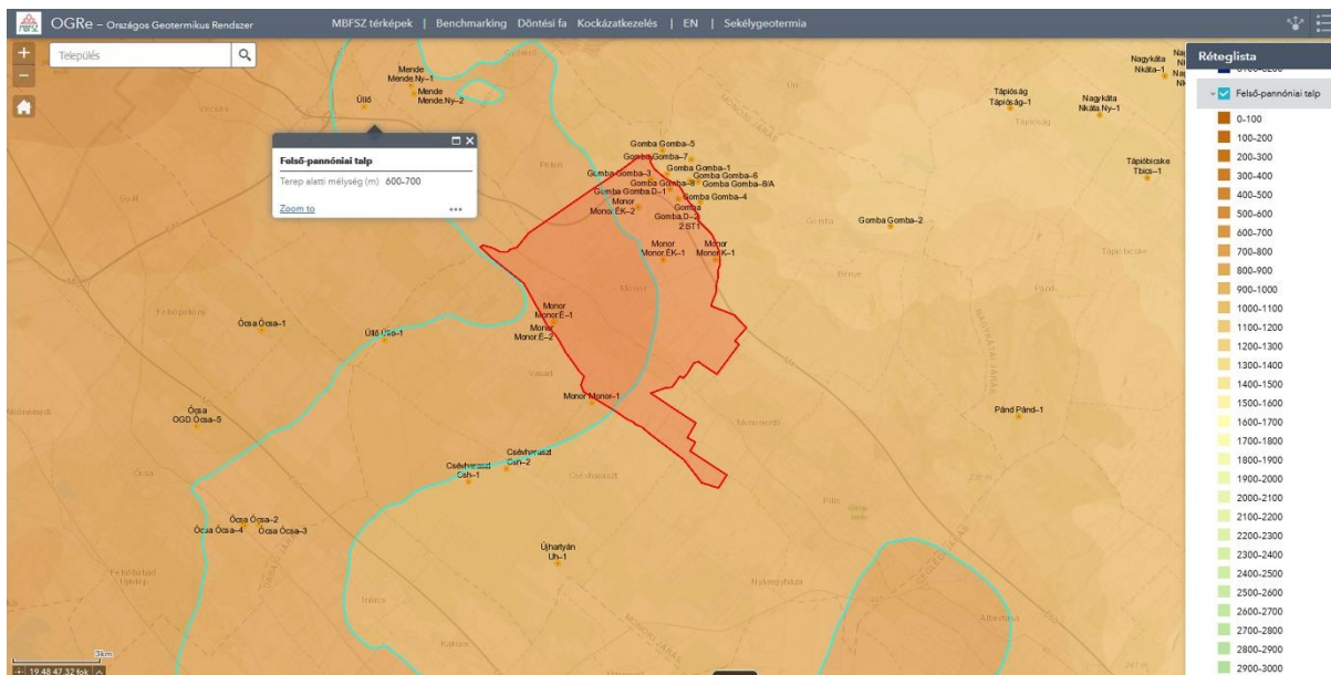
39. ábra A jelentősen jó vizadó rétegeket tartalmazó és leggyakrabban rétegvíz kinyerésre alkalmas, termálvizhasznosításra is megfelelő felső-pannon korú kőzetrétegek talpmélység-térképe Monor környezetében. A talpmélység nyugati irányból kelet és délkelet felé csökken. Mélysége Monor Ny-i részén 600-700 a terepszint felett, míg ez keletebbre kb 100 méterrel feljebb húzódik. (forrás: MBFSZ térképszoftver – SZTFH)
