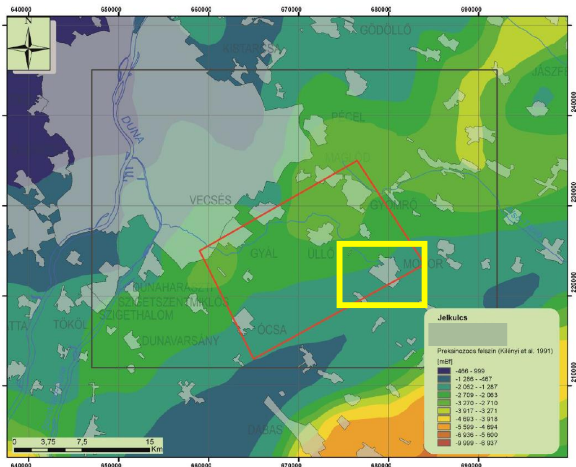
33. ábra Monor környezet prekainozóos medencealjzatának szintvonalas térképe (Kilényi & Sefara 1991). Sárga kerettel jelöltük Monor környezetét
