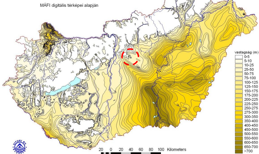
43. ábra Magyarország negyedidőszaki képződményeinek izohipszás vastagság térképe. Monor térsége az Alföld északnyugati peremvidékéhez van közel, amely által a pleisztocén rétegek vastagsága messze elmarad az Alföld belsőbb területeihez képest (szerkesztette: VITUKI Rt, MÁFI digitális térképei alapján)
