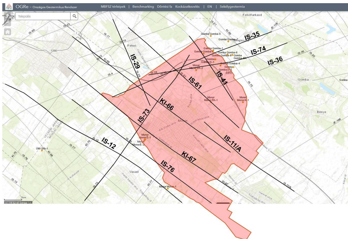
29. ábra Monor földtani és vízföldtani környezetének megismerésében és feltárásában a fúrásokon kívül igen nagy szerepe van a szeizmikus méréseknek. A térkép az eddig elvégzett 2D szeizmikus mérések legfontosabb ismereteket tartalmazó szelvényeit mutatja (forrás: MBFSZ térképszerver – SZTFH)
