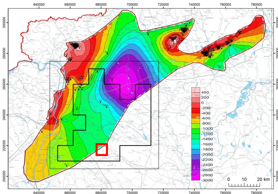
38. ábra Az oligocén Tardi Agyag Formáció talpának tengerszinthez viszonyított mélységtérképe (szerk.: Kercsmár Zs., Uhrin A.) a Magyar Paleogén Medence területén., Piros határolóval jelöltük Monor térségét, ahol a képződmény települési mélysége: ~1400 mBf.
