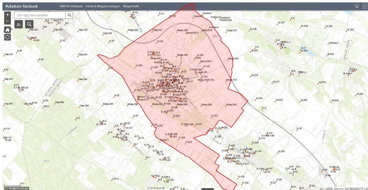
27. ábra Monor területére eső, regisztrált és reambulált földtani ismeretekkel rendelkező fúrások (elérhető adattári fúrások) elhelyezkedése (forrás: MBFSZ térképszerver – SZTFH)
