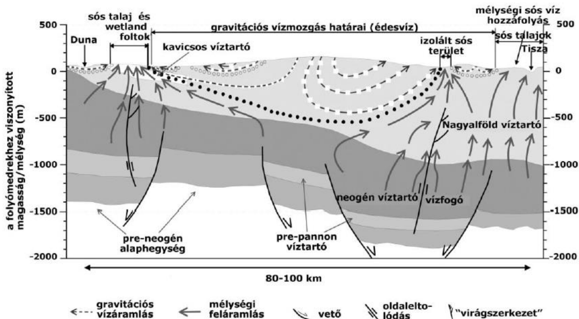
46. ábra A Duna-Tisza köze hidraulikai és vízrétegtani profilja (forrás: Mádlné Szőnyi & Tóth J 2009)
