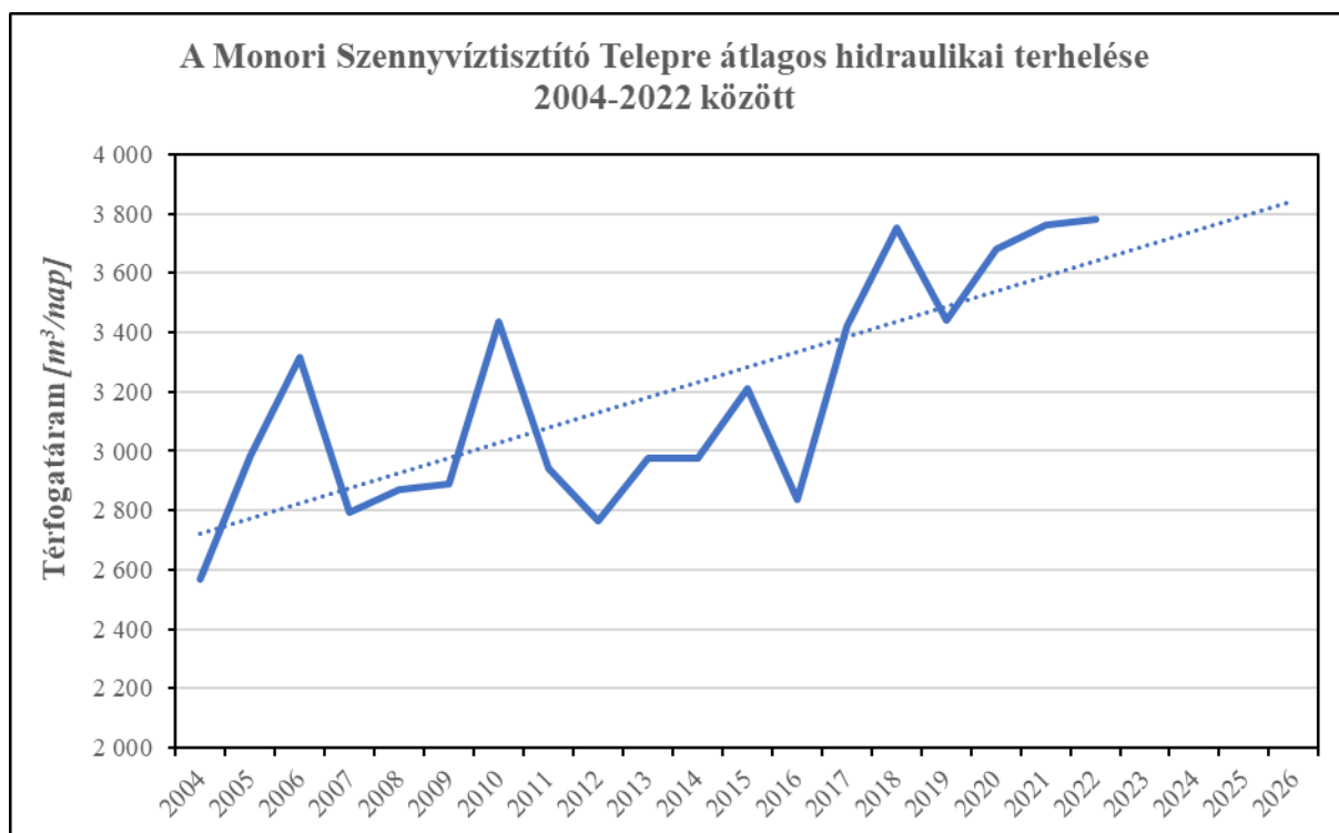
22. ábra: A Monori Szennyvíztisztító Telepen mért befolyó szennyvízmennyiség alakulása [Üzemeltetői adatszolgáltatás]
