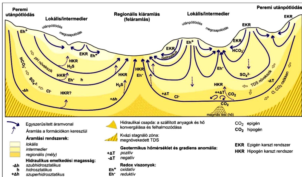
45. ábra Monor földtani környezete kiválóan beilleszthető a Tóth féle egységmedence áramlási rendszerébe. A terület átmenet képez a hegységperemi pozícióból az Alföld irányában érvényesülő, több szintben zajló, mély és sekélyáramlási rendszereket is tartalmazó hidrogeológiai rendszerek között (forrás: Tóth (1999) és Klimchouk (2007) alapján)
