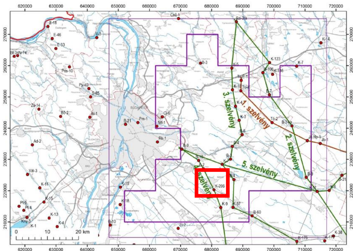
41. ábra A legfelső 200-300 m vastag földtani rétegeket legteljesebben feldolgozó fúrások és azokat érintő szelvények nyomvonala a tágabb vizsgálati térségben. A 4. számú szelvény É-D-i irányban harántolja Monor területét (a Monor K-206 jelű fúráson át), amelyet a következő ábrán részletesebben is bemutatunk (forrás: Monor szénhidrogén koncesszióra javasolt terület komplex érzékenységi és terhelhetőségi vizsgálati jelentése, MBFH, 2014)
