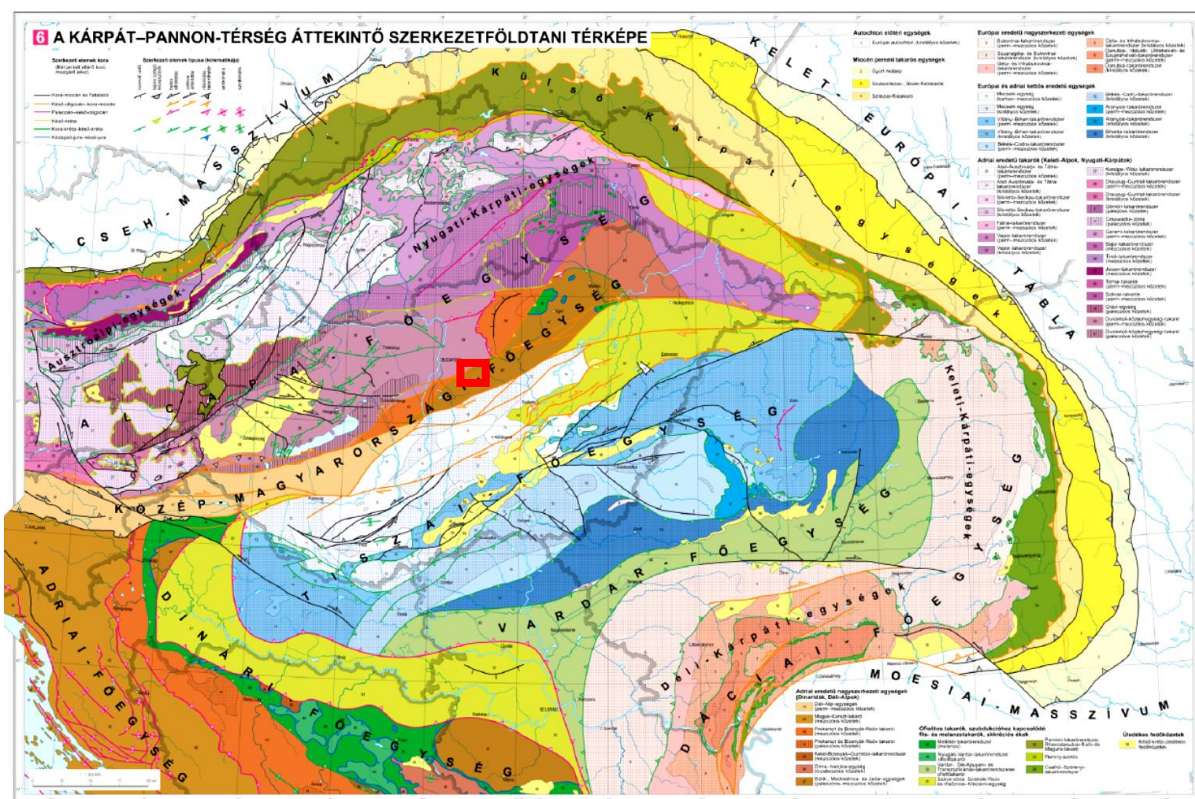
30. ábra Magyarország paleozóos-mezozóos eredetű nagyszerkezeti egységeinek jelenlegi pozíciója. Piros négyzettel jelöltük a Közép Magyarországi Szerkezeti Egység, azon belül a geológiai és hidrogeológiai feldolgozás tárgyát képező Monor földtani környezetét. A terület az azonos nevű szerkezeti főegység része, közvetlenül határon a Dunántúli-középhegységi szerkezeti egységgel. Kettő között található hazánk talán legjelentősebb, elsőrendű törésvonalja a Közép-Magyarországi diszlokációs öv, melynek hely elnevezése: Balaton-Tóalmás vonal (alaptérkép: HAAS et. al. 2014)
