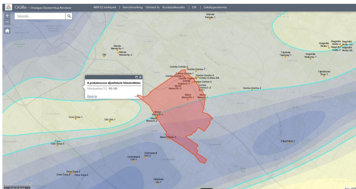
51. ábra A prekainozoos aljzat (felszín)várható közethőmérséklete Monor térségében. A legkedvezőbb esetben a 90-100 °C-os izohipsza húzódik a közigazgatási terület északi felén, míg délre a medencealjzat emelkedésével együtt rohamosan csökken a medencealjzat felületének várható közethőmérséklete is (forrás: MBFSZ térképszerver – SZTFH)
