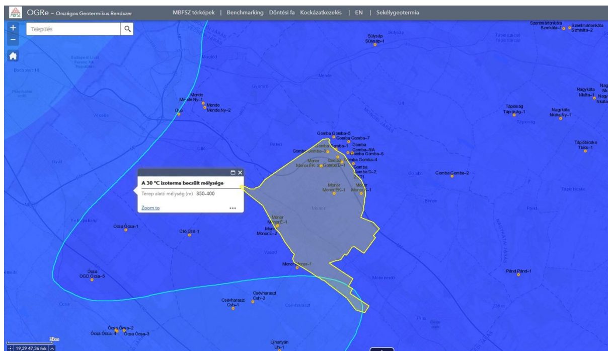
50. ábra A 30 °C-os izoterma mélységi lefutása Monor térségében. A 30 °C terepszint alatti 350-400 m mélységben várható (forrás: MBFSZ térképszerző – SZTFH)
