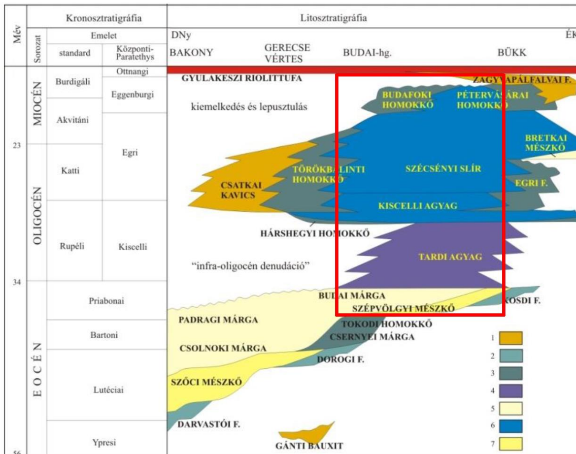
37. ábra A paleogén üledékciklus litosztratigráfiai (közetrétegtani) és faciológiai összefüggései a Magyar Paleogén medencében (Tari et al 1993 alapján)
