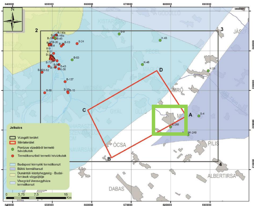
48. ábra A 30 °C-nál magasabb hőmérsékletű kifolyó vizet adó kutak térképe a vízadó képződmények kora alapján leválogatva. Zöld kerettel jelöltük Monor környezetét
